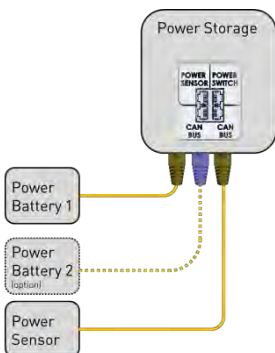
Zusätzliche Power Sensor Kommunikation
