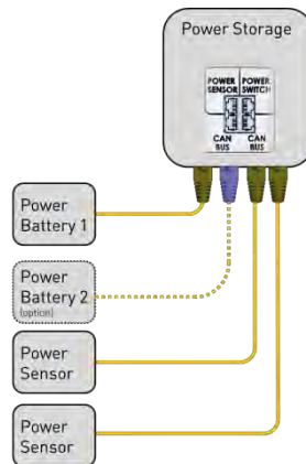
Zusätzliche Power Switch Kommunikation
