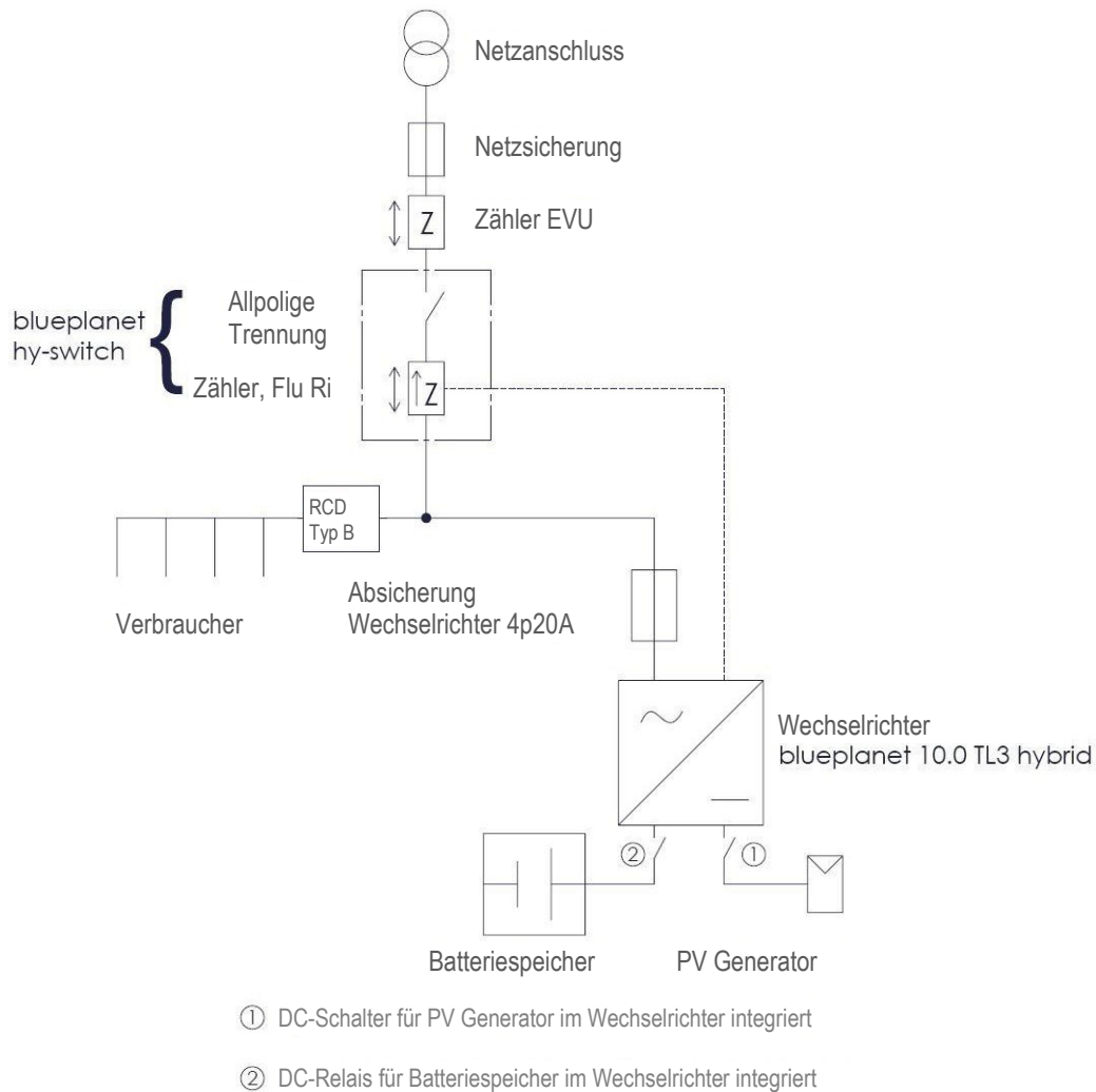
Abb. 1: Schema der Anlage. Bei Inselssystemen entfällt der Pfad Netzanschluss bis blueplanet hy-switch
