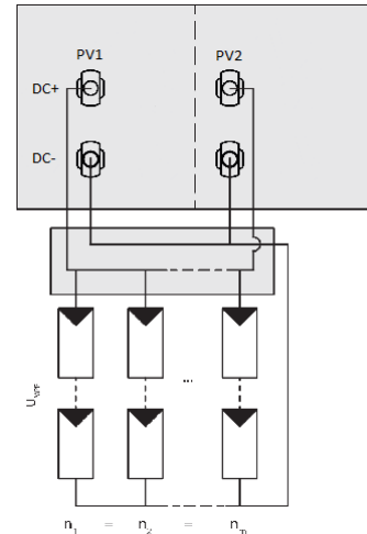
Abb. 24: Parallele Eingangsbeschaltung für ein oder mehrere Modulstränge.
