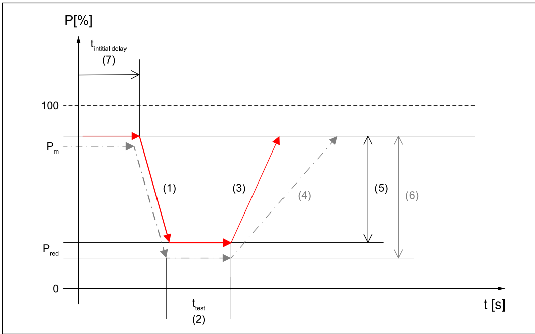
Anwendungsbeispiel mit „Return Gradient 1 Alternative“ und „Return Gradient 1 Alternative Threshold“.
