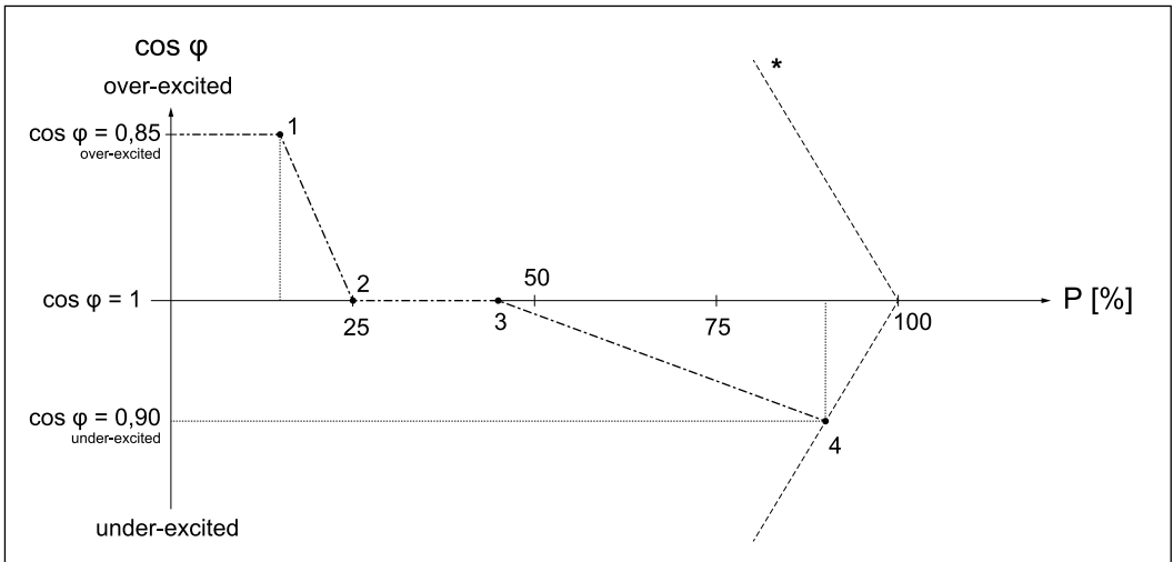
Beispiel: Kurve durch 4 Stützpunkte definiert.
