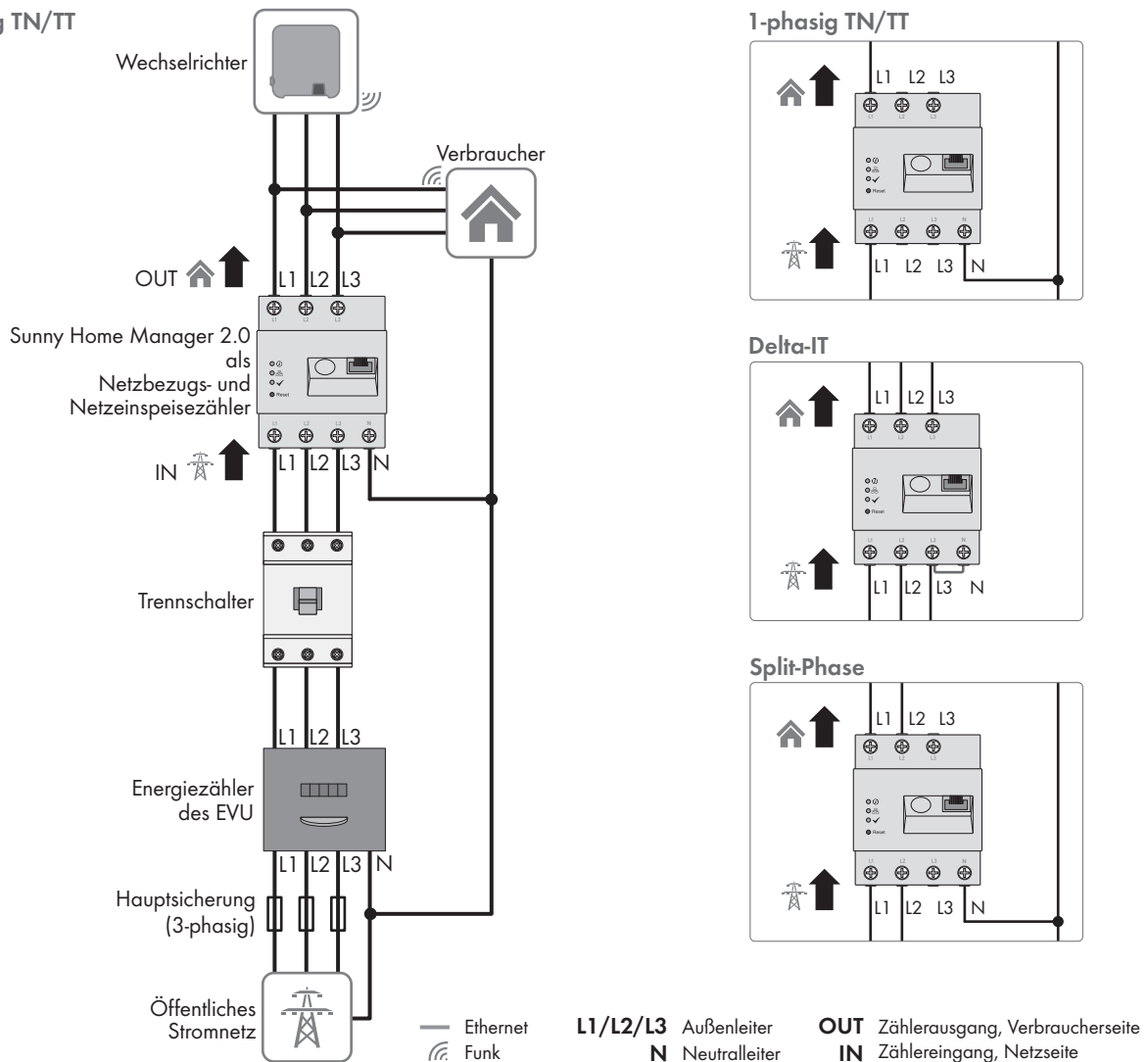
Abbildung 5: Anschlussbeispiel in TN- und TT-Stromnetzen bei Installation am Netzanschlusspunkt unter Verwendung der integrierten Messeinrichtung
