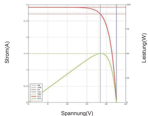
RNG-50DB-H Eigenschaften gegen Spannung
